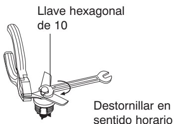
Desmontaje cuchilla
